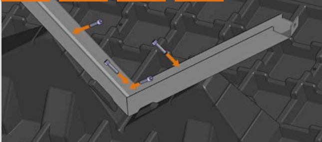
3 Knick-Fix-Winkel in den Grundplatten befestigen
