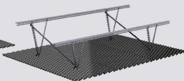
4 Modulträger-Profile und Diagonalprofile montieren
